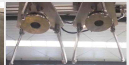
Garra especial para baldes de boca larga
